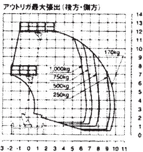
●作業範囲図
