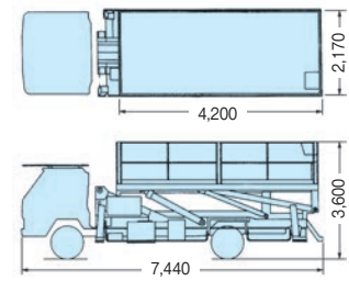
●車両寸法図
