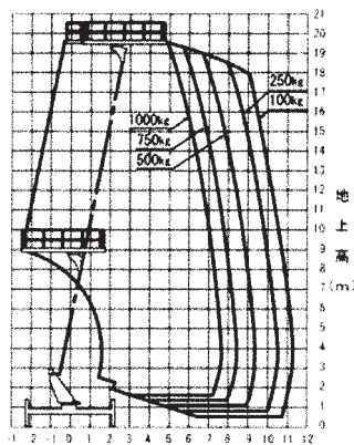
●作業範囲図
