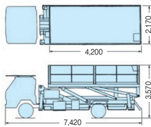
●車両寸法図
