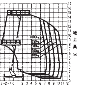
●作業範囲図
